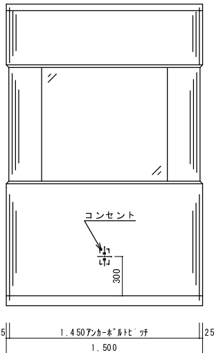
A 立面図
