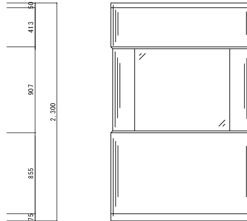
C 立面図
