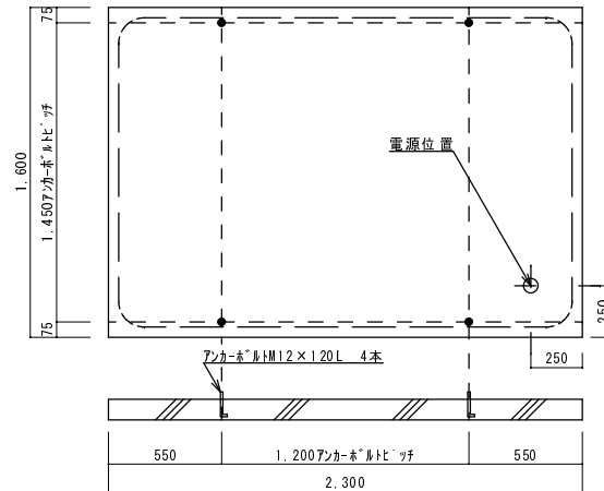
基礎図 (参考)
