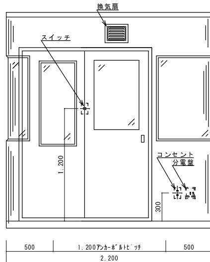
B 立面図
