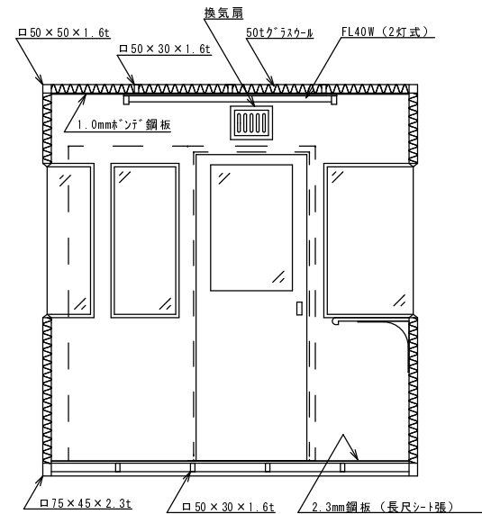
D-D 立面図
